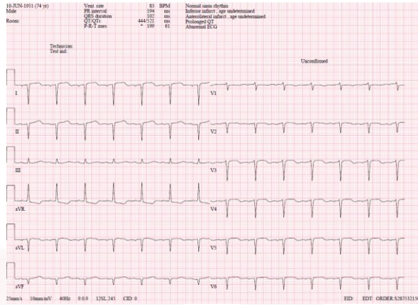
Dekstrokardi EKG
