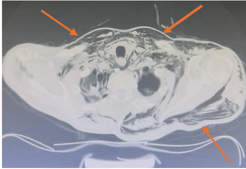
Pnömotoraks (PX)
