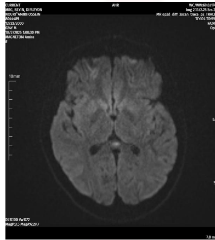
difüzyon mr
